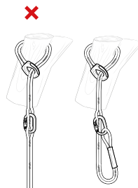
6.5 falsche Anwendung der Zwischennähte Incorrect use of intermediate seams
