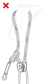
6.1 Ring auf Kausche -> erhöhter Verschleiß Ring on thimble -> increased wear
