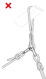
6.2 Der Ring und seine Schlinge dürfen nicht in verschiedene Richtungen belastet werden The ring and its sling must not be loaded in different directions
